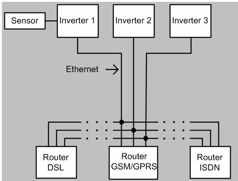
Abb.: 1 Beispiele zur Vernetzung von 3 REFUSOL Wechselrichtern mit dem Überwachungsportal REFULOG
